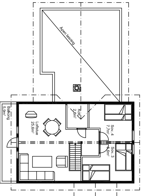
Loftsplan
