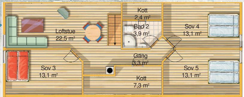
Loftsplan
